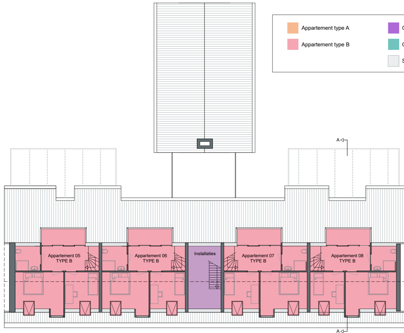
Verdieping 2 (+9865)
