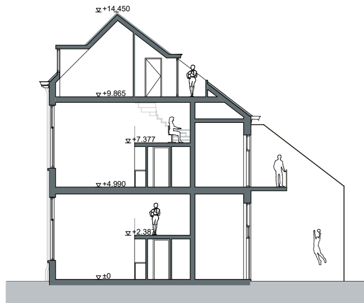
Doorsnede A-A
