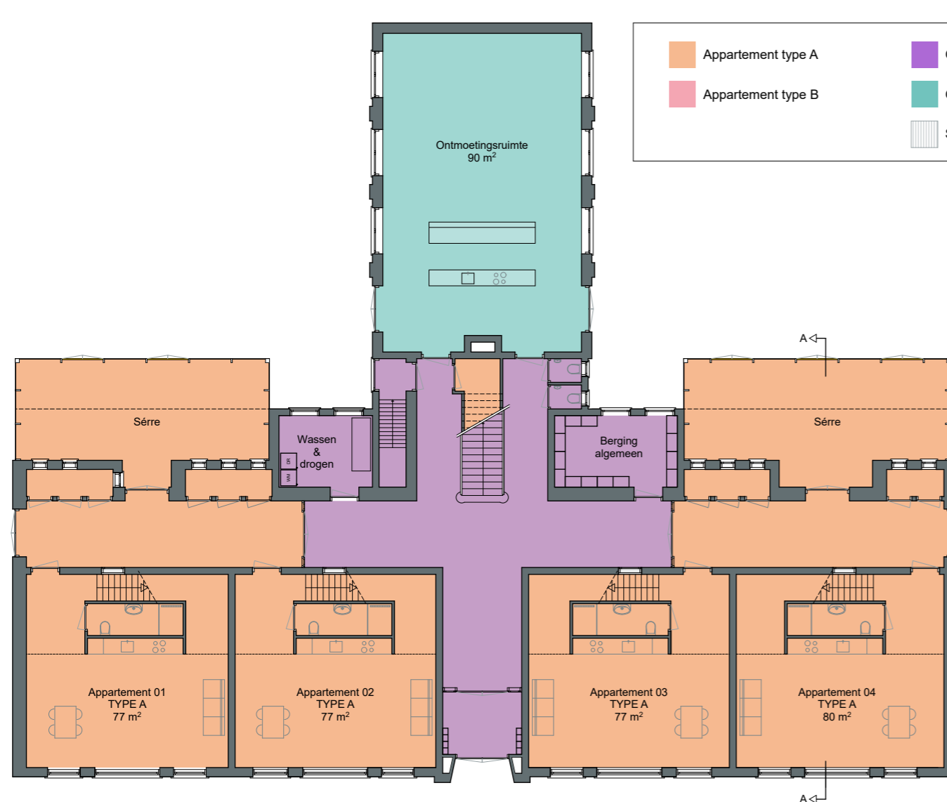
Begane grond (Peil=0)
